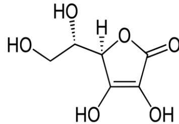
Vitamine C C_6H_8O_6
