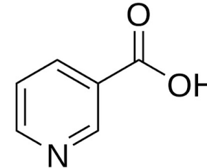
Vitamine B3 (Niaminacide) C_6H_5NO_2
